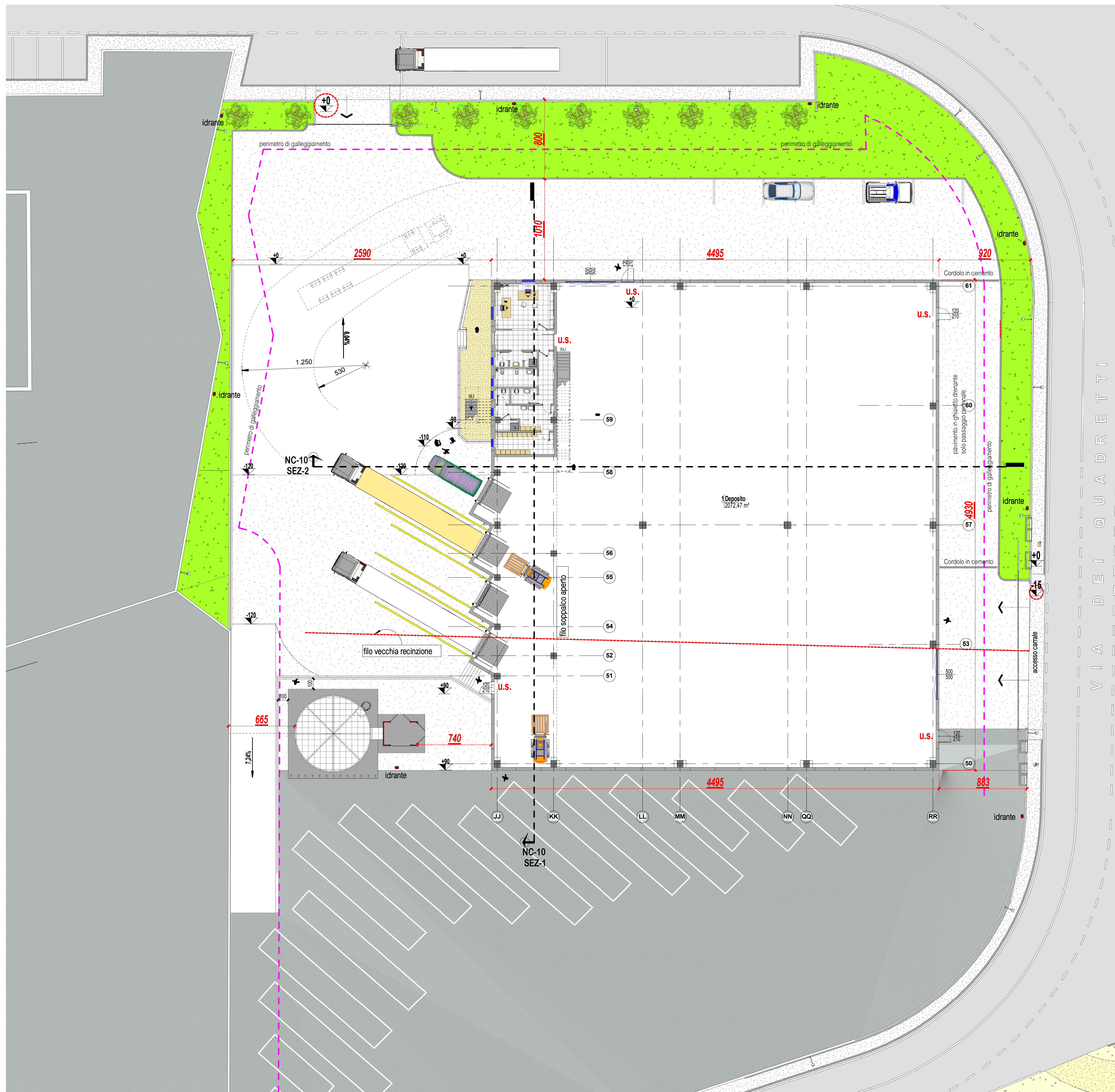
NC-PLANIMETRIA GENERALE 1:200
