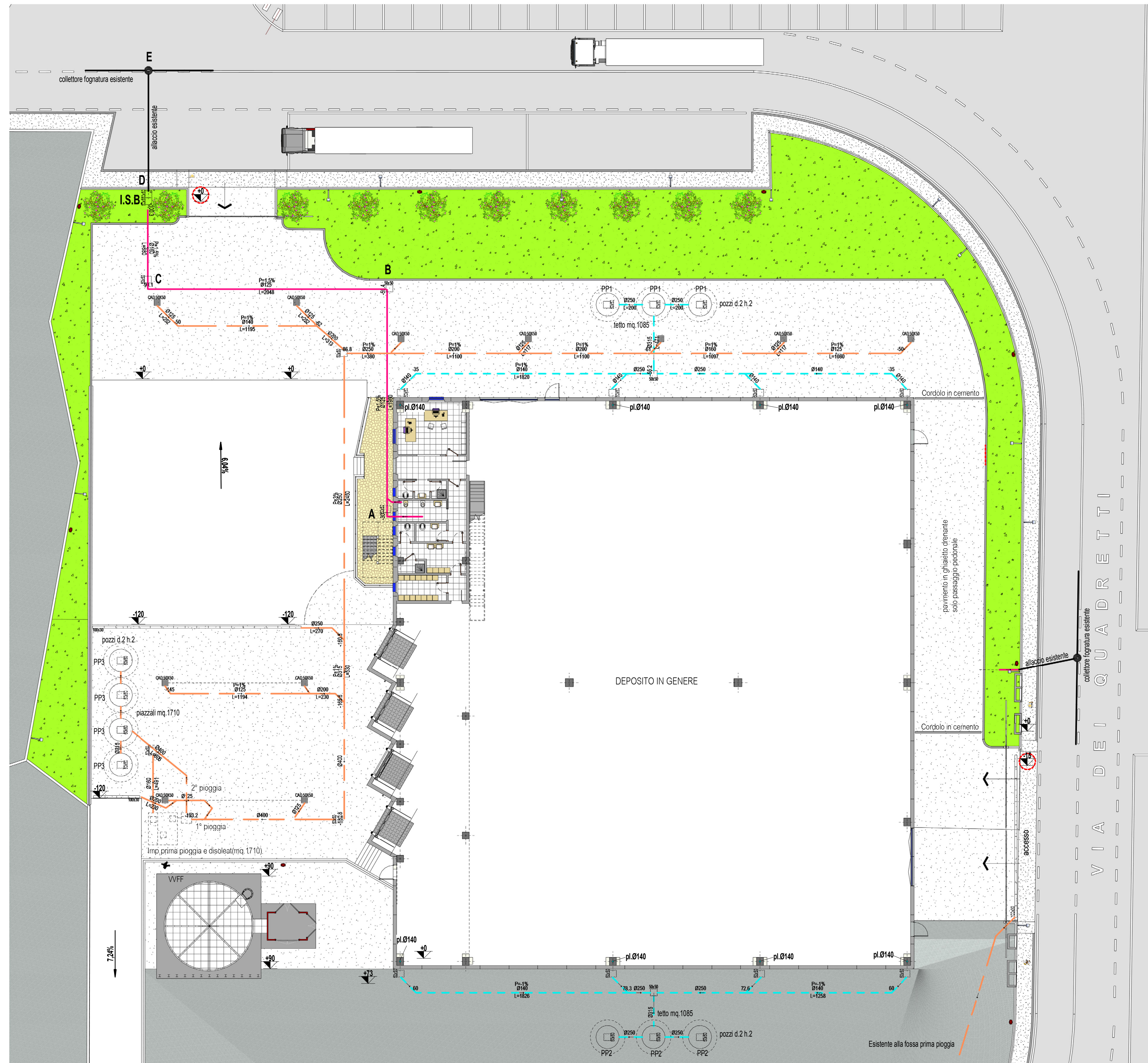
NC-SCHEMA PLANIMETRIA FOGNATURA (Cogeide) T. 200
