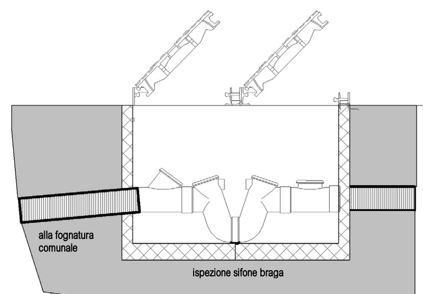
NC-DETTAGLIO POZZETTO T. 20
