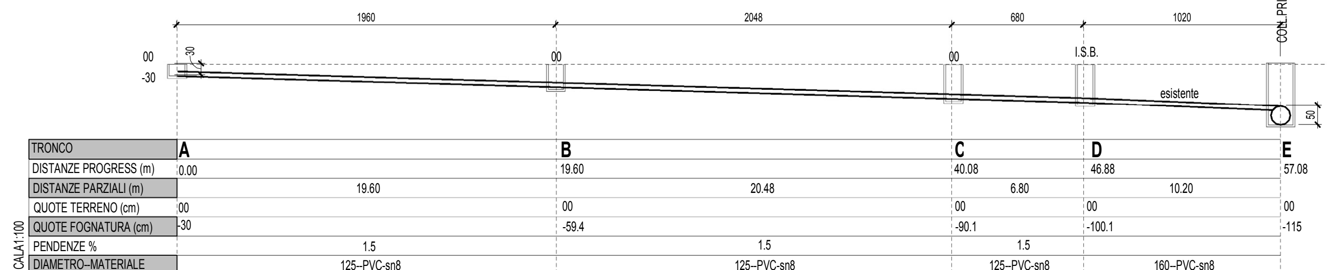
NC-SEZIONE FOGNATURA Acque nere
